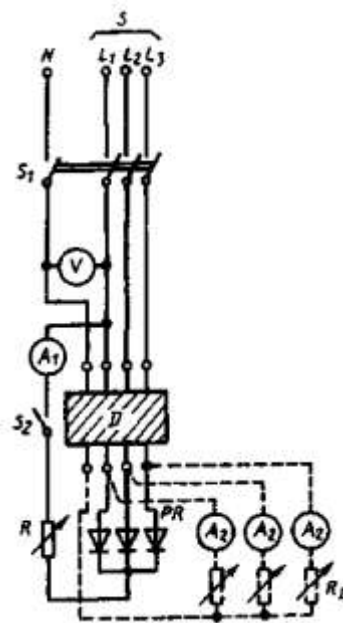
A_1 — амперметр действующих значений; A_2 — амперметр постоянного тока; D — испытуемое УЗО — Д; PR — трехфазное однополупериодное или двухполупериодное соединение; R — регулируемый резистор для дифференциального тока; R_L — активная нагрузка; S — источник питания переменного тока; S_1 — многополюсный выключатель; S_2 — однополюсный выключатель; V — вольтметр
