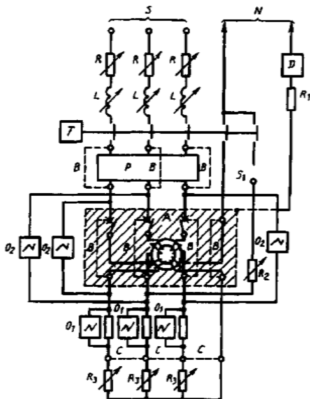
N — нулевой провод; S — источник электрической энергии; R — регулируемый резистор; L — регулируемая катушка индуктивности; P — аппарат защиты от коротких замыканий; B — временные соединения для калибровки; C — соединения для испытания при номинальном условном токе короткого замыкания; T — устройство, создающее короткое замыкание; O_1 — самописец, регистрирующий ток; O_2 — самописец, регистрирующий напряжение; D — детектор обнаружения аварийного тока повреждения; R_1 — резистор, ограничивающий ток в устройстве D ; R_2 — регулируемый резистор для калибровки тока отключения I_{\Delta} ; R_3 — дополнительный регулируемый резистор для получения токов меньших по величине номинальных условных токов короткого замыкания; S_1 — вспомогательный выключатель; A — УЗО — Д, подвергаемое испытанию
