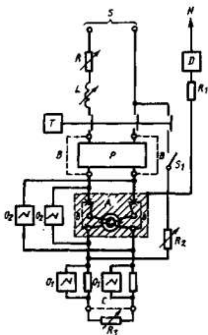
Рисунок 6 — Схема испытательной цепи для проверки правильной координации с аппаратом защиты от коротких замыканий и номинальной включающей и отключающей способности двухполюсного УЗО — Д без встроенной защиты от коротких замыканий в однофазной цепи
