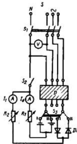
S — источник электрической энергии; I — независимая линия питания; V — вольтметр; A — амперметр; D — УЗО — Д, подвергаемое испытанию; Di — диоды; R_1 и R_2 — регулируемые резисторы; S_1 — многополюсный выключатель; S_2 — однополюсный выключатель; S_3 — двухполюсный выключатель на два направления; S_A — вспомогательный выключатель
