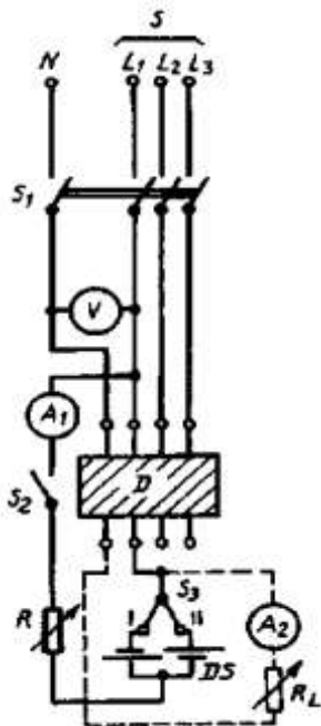
A_1 — амперметр постоянного тока; A_2 — амперметр переменного тока; D — испытуемое УЗО — Д; D_s — источник постоянного тока; R — регулируемый резистор; R_L — активная нагрузка; S — источник питания переменного тока; S_1 — многополюсный выключатель; S_2 — однополюсный выключатель; S_3 — двухполюсный выключатель на два направления; V — вольтметр
