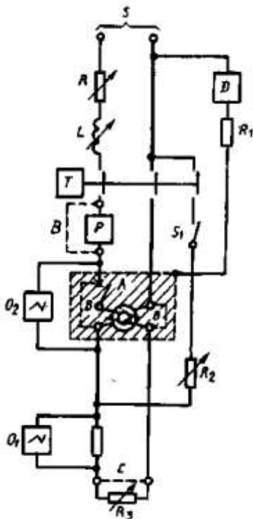
Рисунок 3i — Испытательная цепь для проверки правильности отключения УЗО — Д в случае медленно повышающегося дифференциального тока в результате повреждения цепи, имеющей двухполупериодную мостовую схему на линейном напряжении
