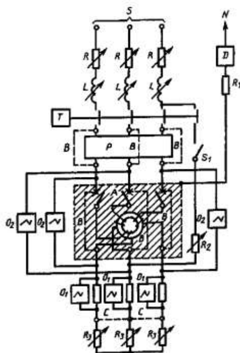
Рисунок 8 — Схема испытательной цепи для проверки правильности координации с аппаратом защиты от коротких замыканий и номинальной включающей и отключающей способности трехполюсного УЗО — Д без встроенной защиты от коротких замыканий в трехфазной цепи
