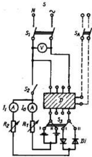
S — источник электрической энергии; I — независимая линия питания; V — вольтметр; A — амперметр; D — УЗО — Д, подвергаемое испытанию; Di — диоды; R_1 и R_2 — регулируемые резисторы; S_1 — многополюсный выключатель; S_2 — однополюсный выключатель; S_3 — двухполюсный выключатель на два направления; S_A — вспомогательный выключатель
