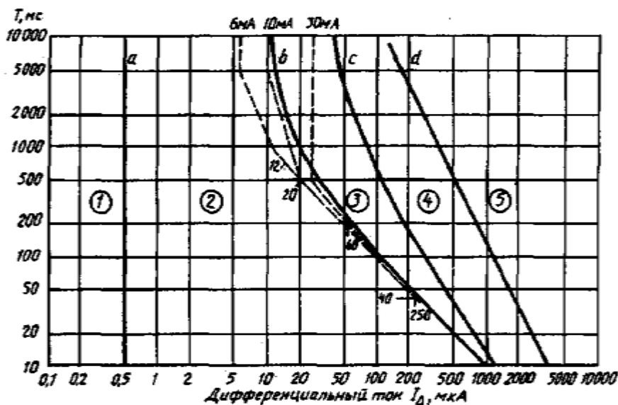
Рисунок 1 — Рабочие характеристики УЗО — Д, дополняющие таблицу III стандарта и сопоставляемые при максимальной длительности напряжения контакта
